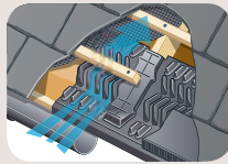
RedVent EavesVent
